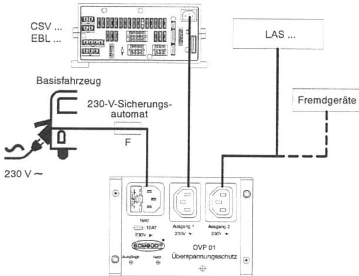
Überspannungsschutz OVP 01 A
